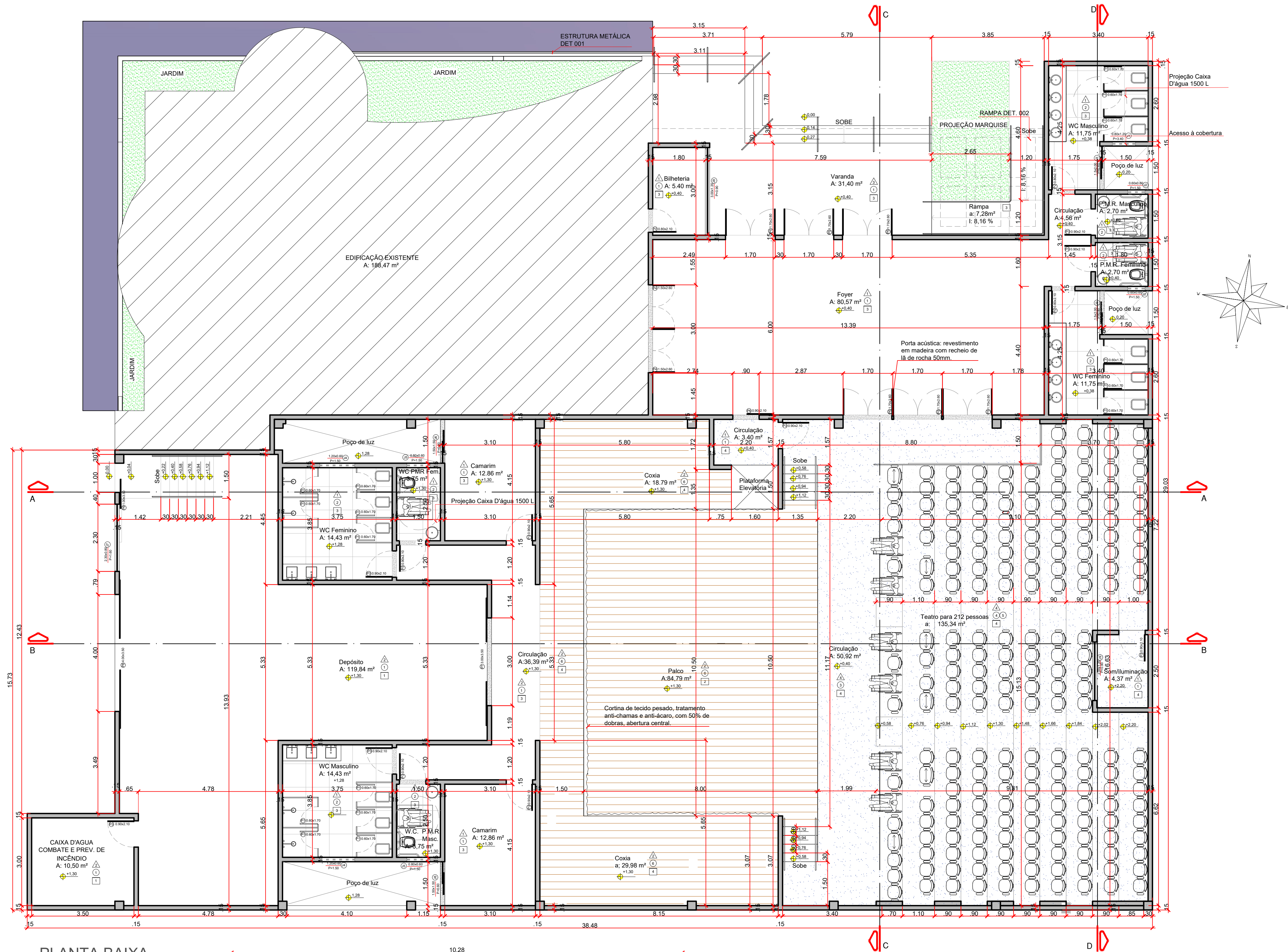
PLANTA BAIXA
