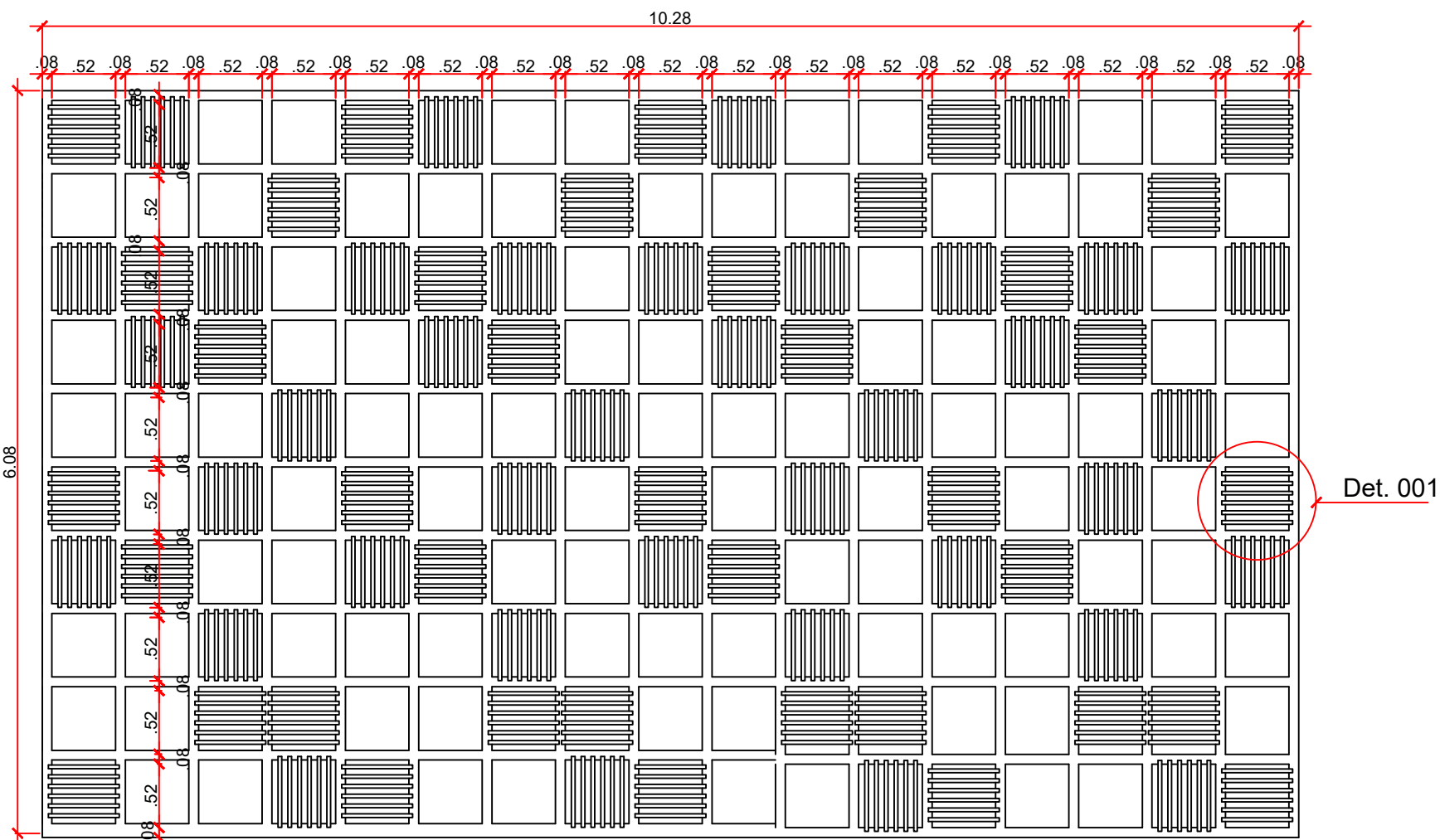
BRISE FRONTAL ESC.: 1/50
