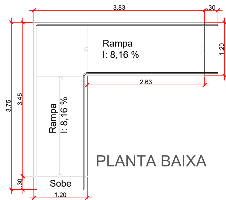
RAMPA DET. 002 ESC.: 1/50
